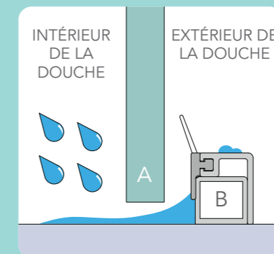
A - Porte coulissante en verre B - Seuil minimaliste I - Joint de seuil
