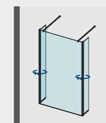
CONFIGURATION 17 – Panneau fixe x1 – Barre de stabilisation droite x2 – Panneau rotatif x2
