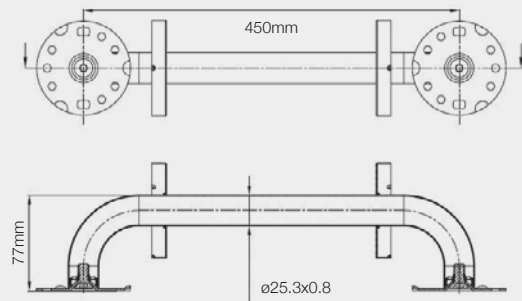
BARRE DROITE DE MAINTIEN 450MM DIAMÈTRE 25MM
