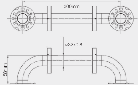
BARRE DROITE DE MAINTIEN 300MM DIAMÈTRE 32MM
