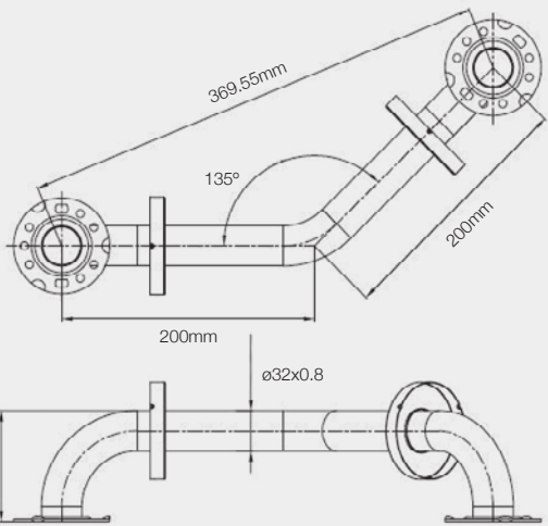
BARRE DE MAINTIEN EN ANGLE 450MM DIAMÈTRE 32MM
