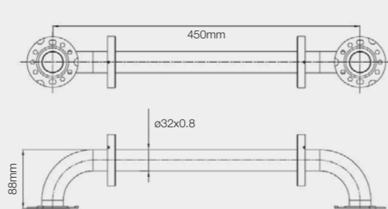
BARRE DROITE DE MAINTIEN 450MM DIAMÈTRE 32MM
