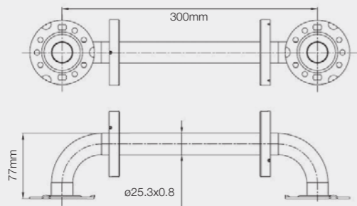
BARRE DROITE DE MAINTIEN 300MM DIAMÈTRE 25MM
