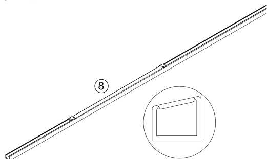
L=1989mm SECH28 Joint magnétique A
