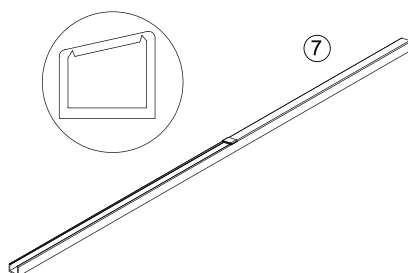
L=1989mm SEFL18 Joint magnétique B
